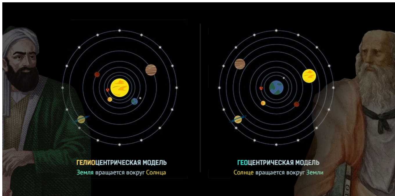
Сравнение гелио и гео центрических моделей
